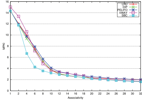
(b) ammp
