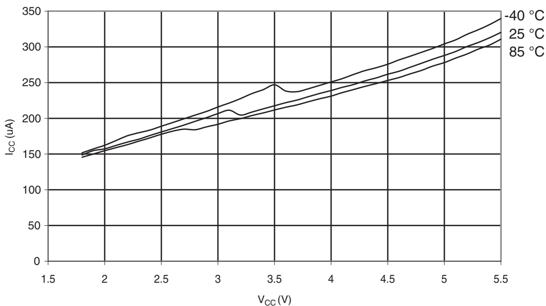
Figure 30-369. ATmega328P: ADC Current vs. V CC (AREF = AV CC )
