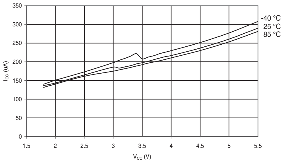
Figure 30-40. ATmega48A: ADC Current vs. V CC (AREF = AV CC )
