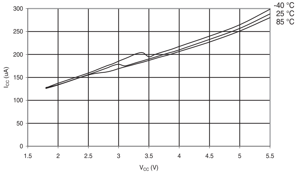
Figure 30-181. ATmega88PA: ADC Current vs. V CC (AREF = AV CC )
